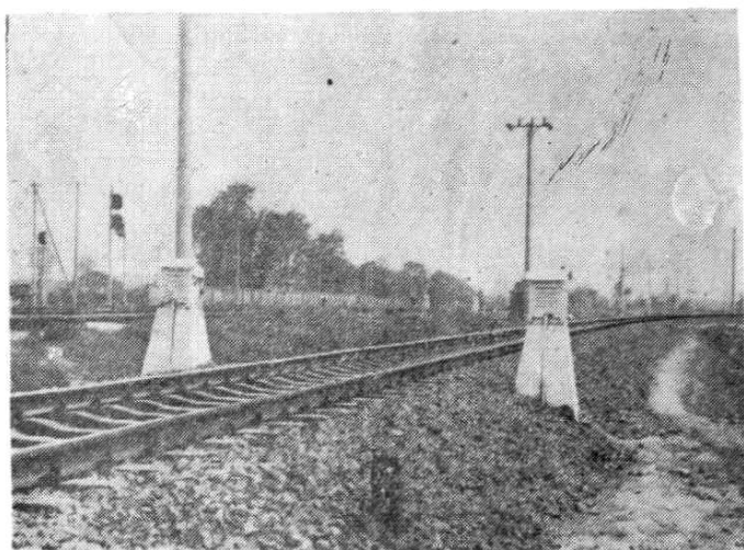
新乡列检红外线轴温探测仪
