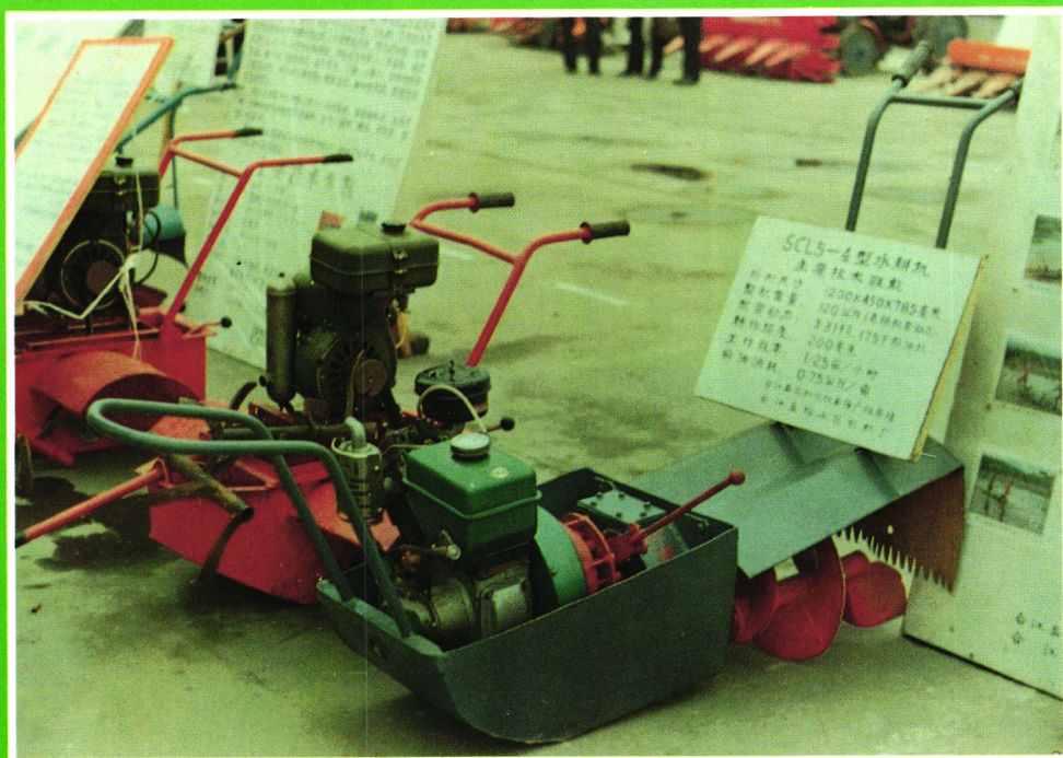
▲威远县共华微型水耕机厂创制的双轴差距螺旋水耕机于1988年10月获中华人民共和国实用新型专利证书
