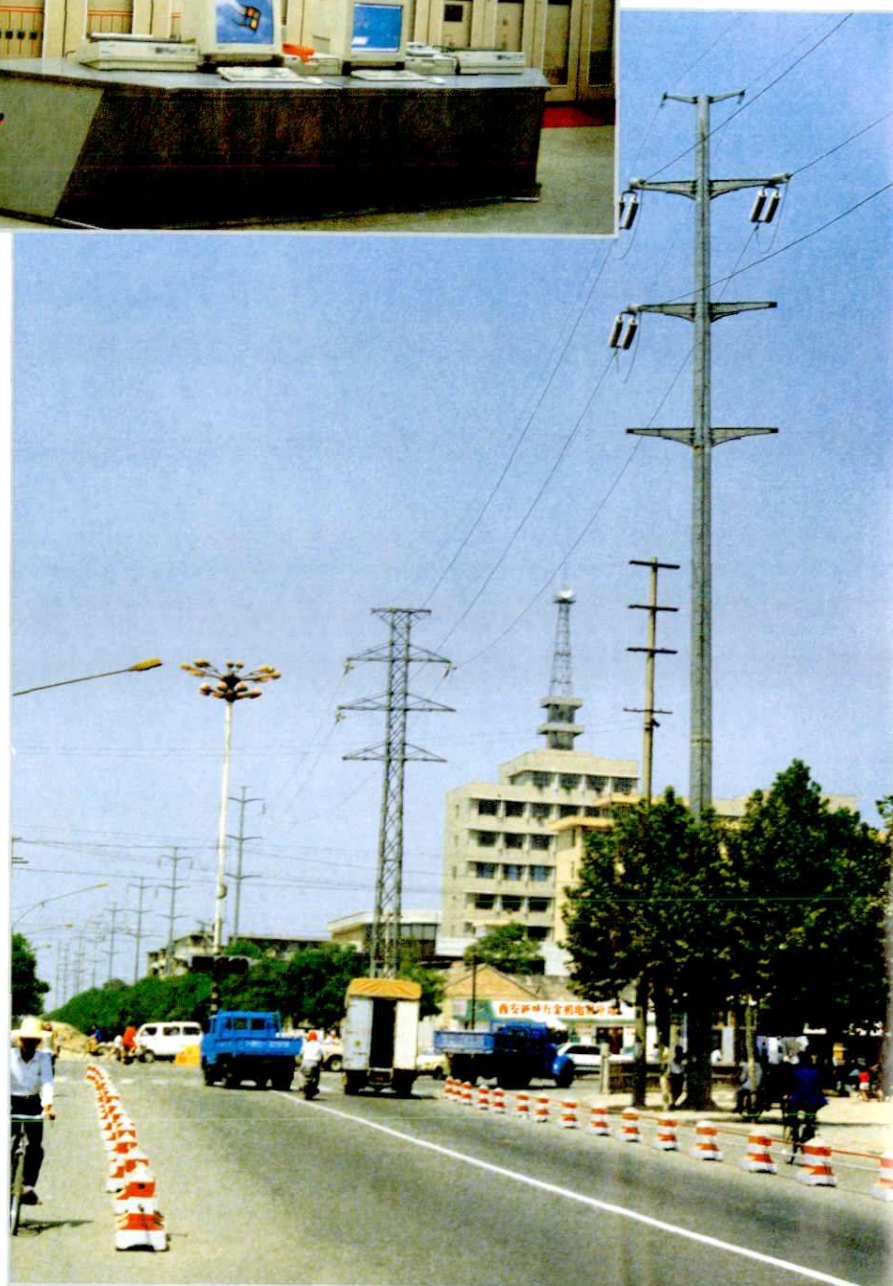
西安城区110千 伏钢管窄基塔
