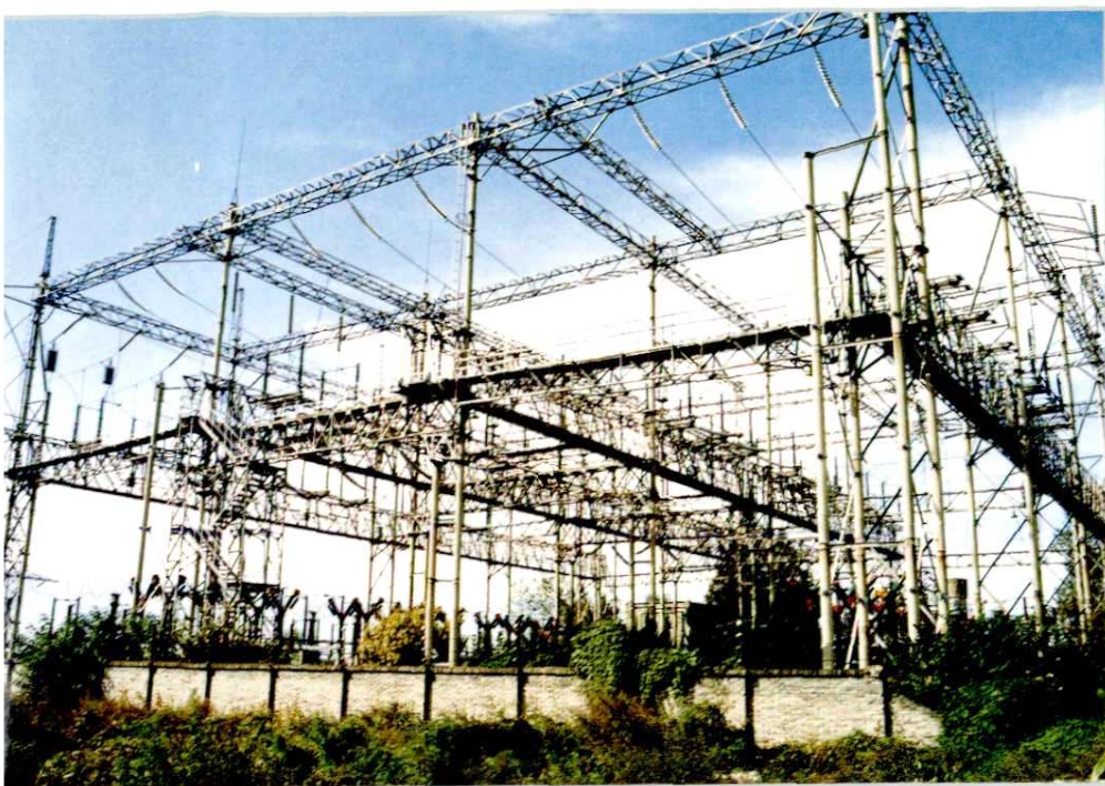
高层布置的 220千伏周至变电站 户外设备区
