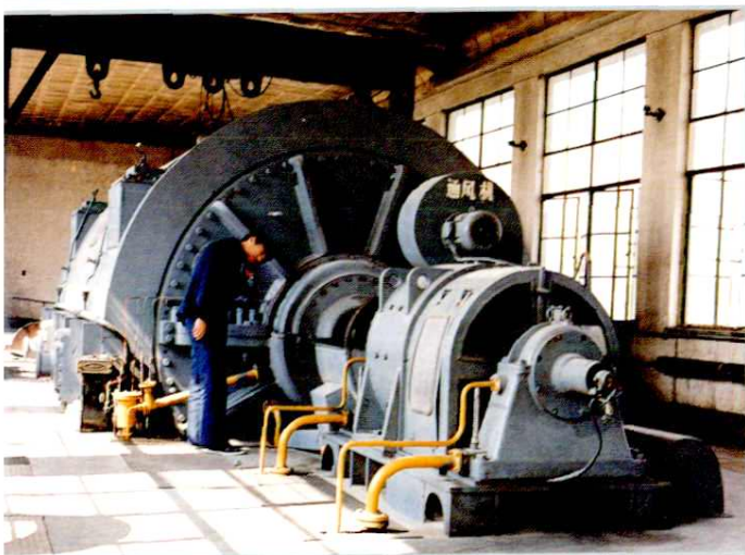
220千伏阎良变电站6万千乏调相机
