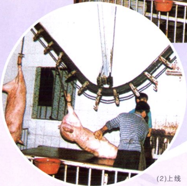
机械化定点屠宰生猪生产线（1999年12月摄）
