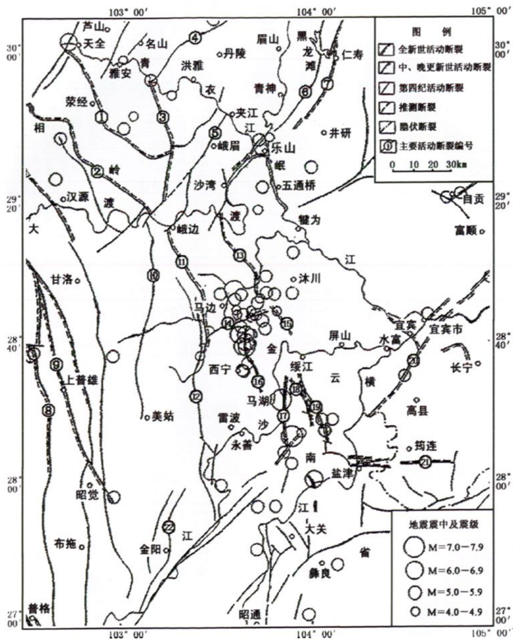
乐山市及邻区地质构造纲要及震中分布图
