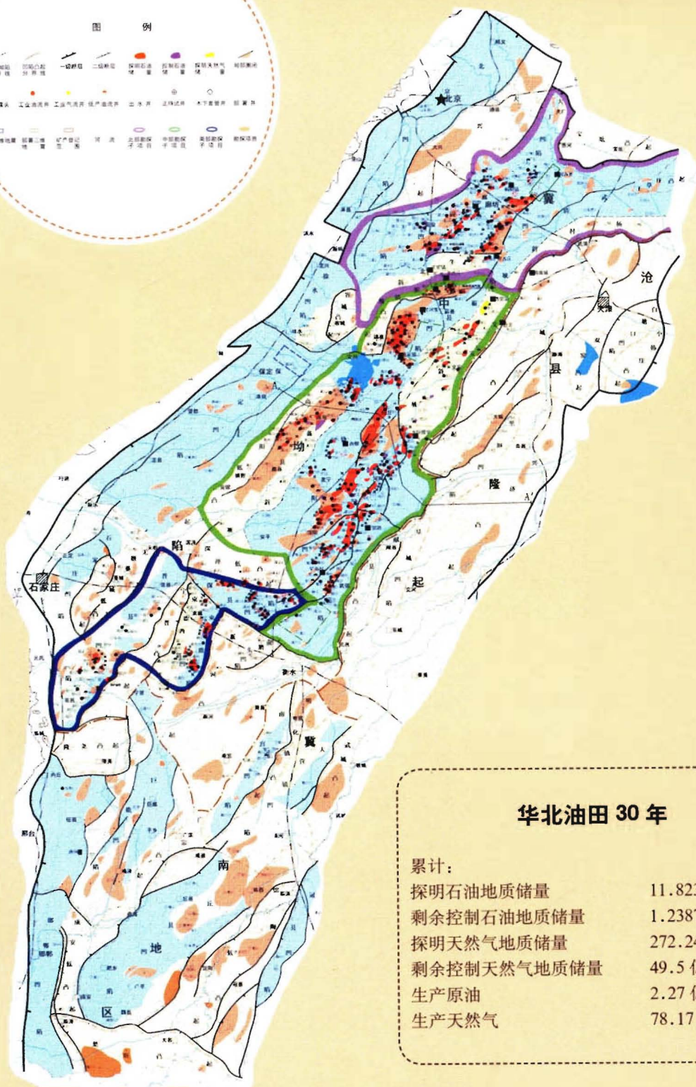
冀中油气勘探形势图
