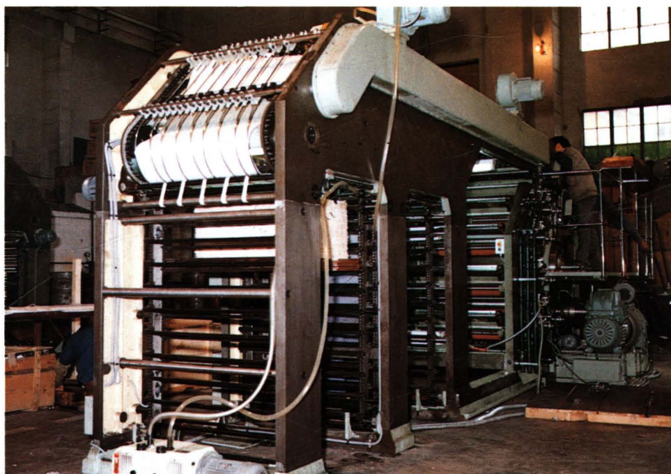
正在运行走纸的 四色轮转凹印机(82型)
