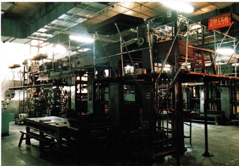
厂生产制造的四色轮转凹印机(72型)
