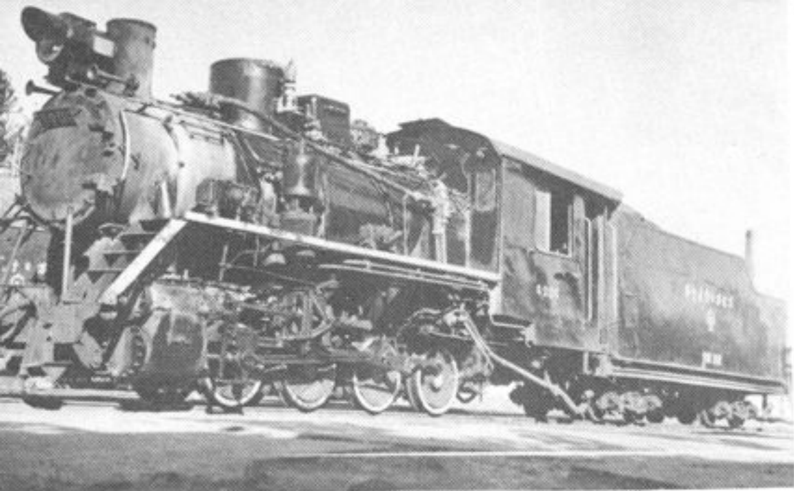
地方铁路42吨蒸汽机车
