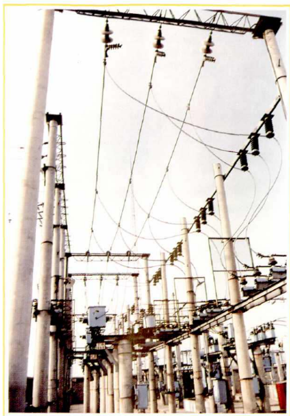
孙吉 110 千伏变电站
