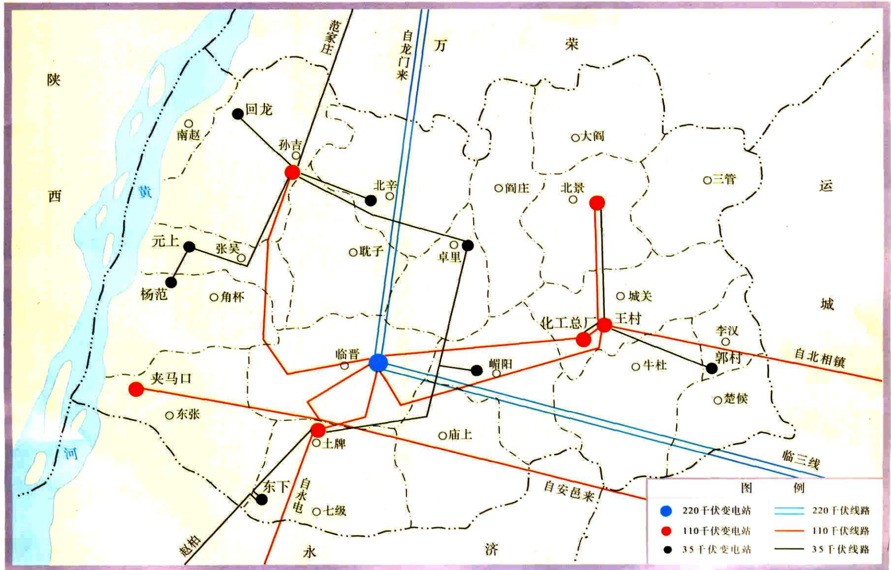
临猗县电力网络地理接线示意图
