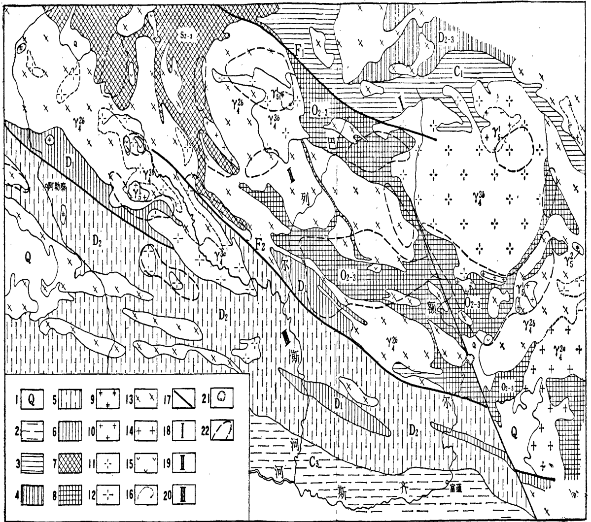
图1-1 阿尔泰中段地质略图
