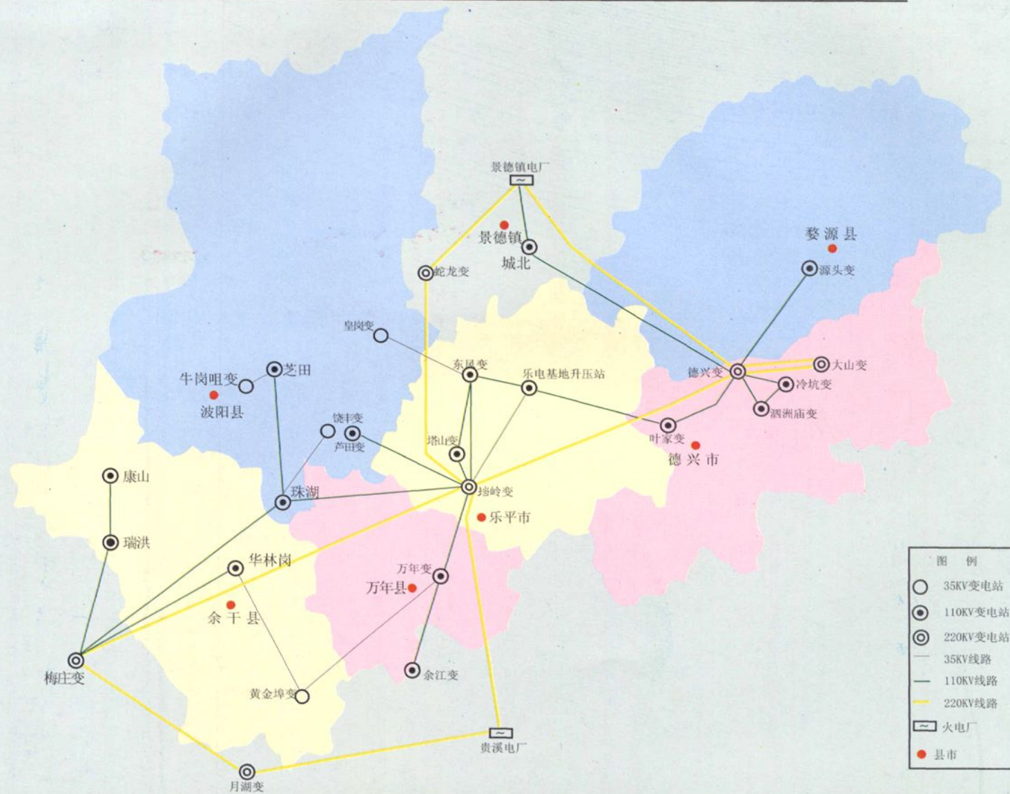
赣东北供电地区电力系统地理结线图（2000年）
