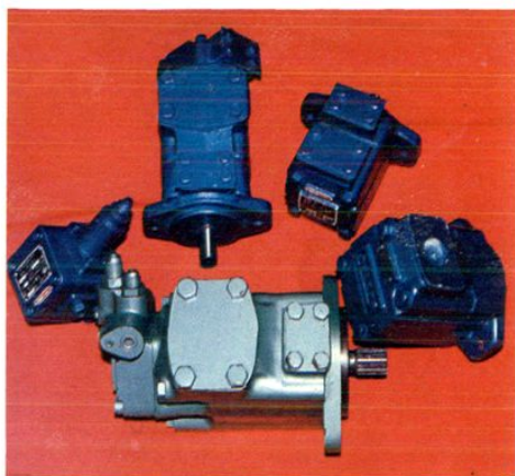
获省部优产品称号的中高压子母式叶片泵
