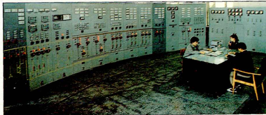
三家庄 220 千伏变电站主控制室。
