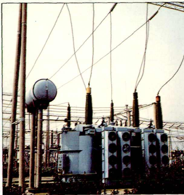
新绛变电站 9 万千伏 安主变压器。
