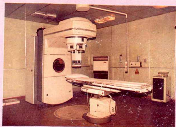
医用直线加速器
