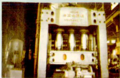
自制设备—1650吨大型 水压机
