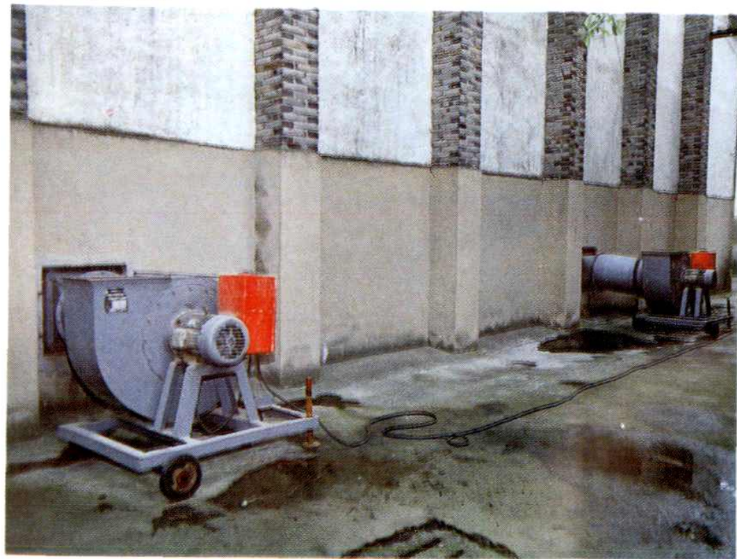
粮仓机械化通风
