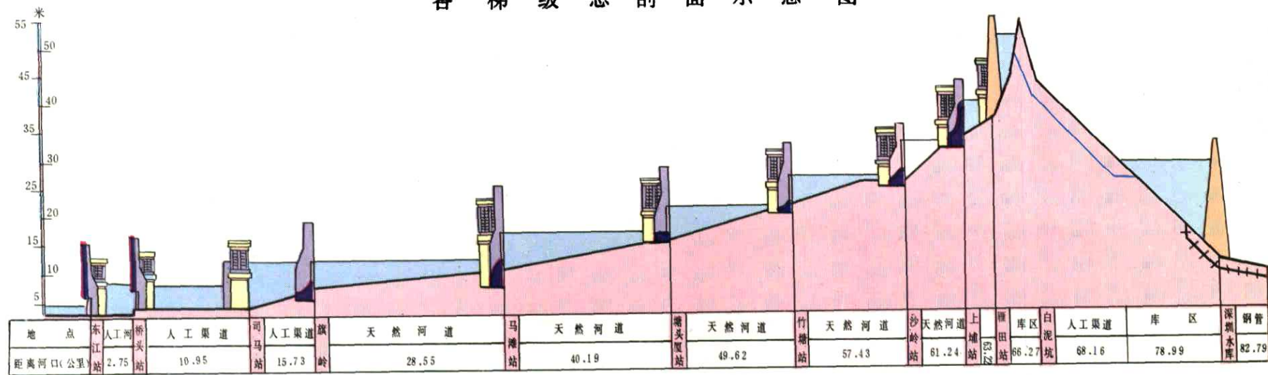
东江 — 深圳供水工程 各梯级总剖面示意图
