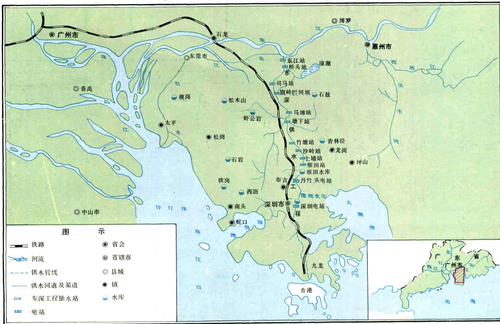
东—深供水工程布置示意图
