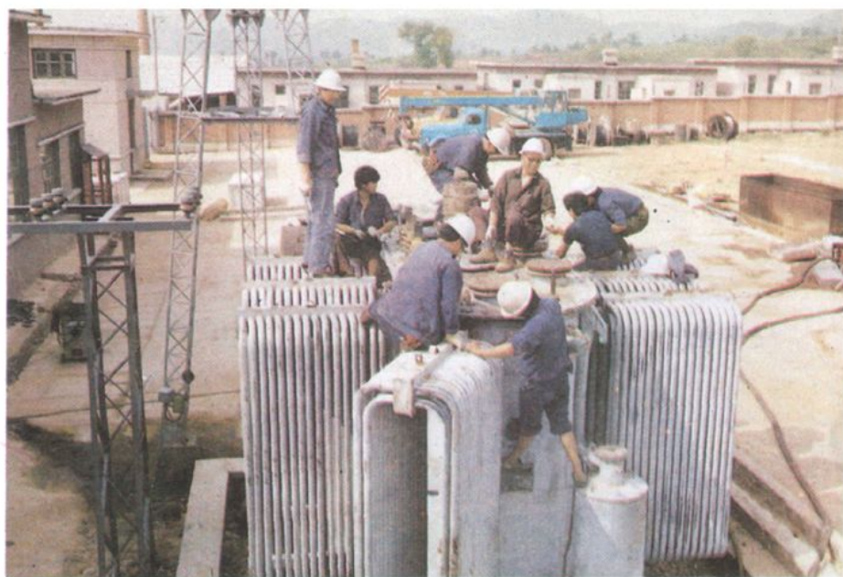
安装公司变电队工人在安装变压器
