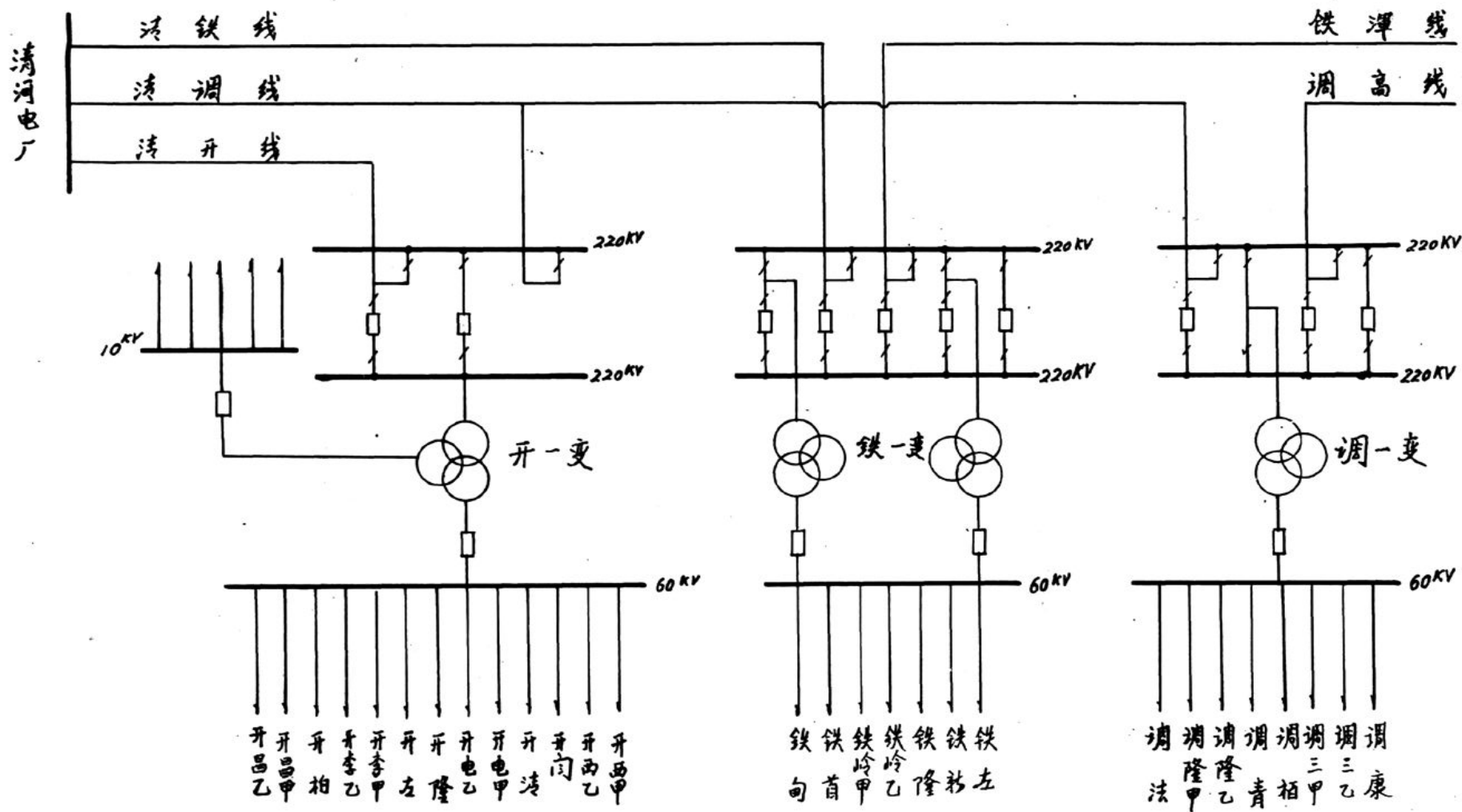
一九八五年铁岭地区220KV系统结线图
