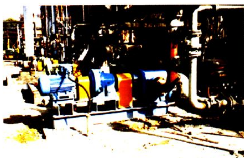
高粘度齿轮泵在使用现场
