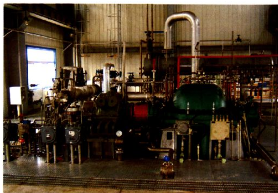
院第一台干气密封产品应用于镇海炼油厂
