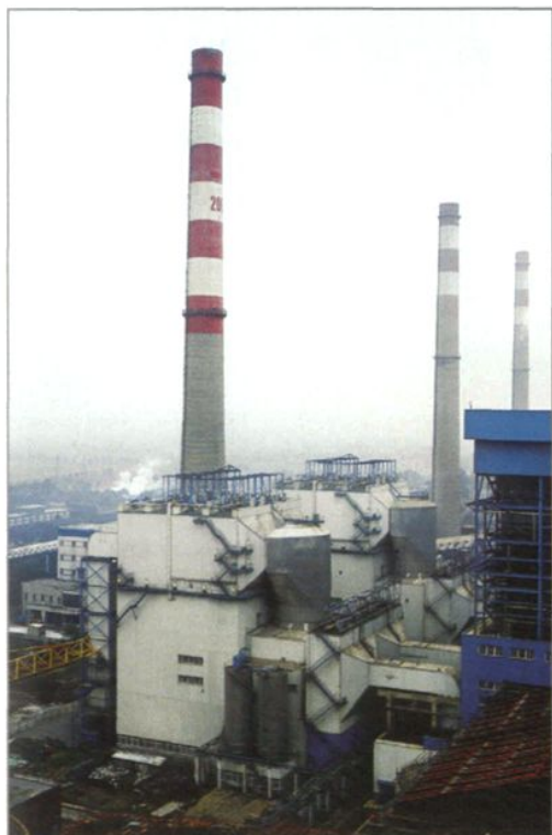
漳山电厂三期干法脱硫工程
