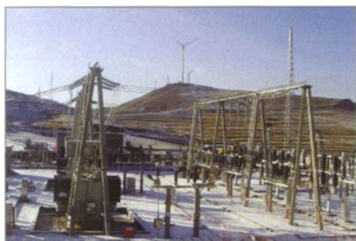
山西宁武风电升压站工程
