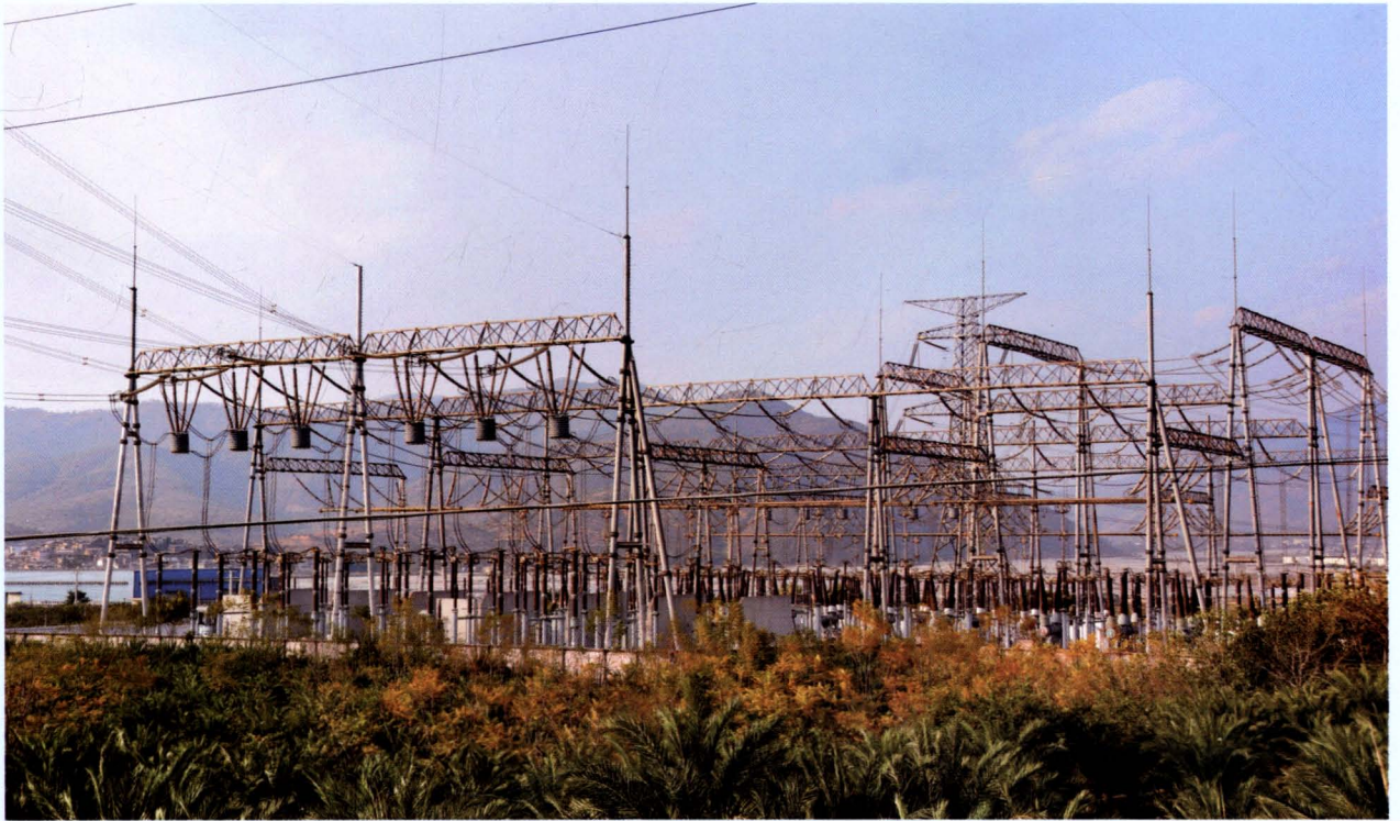
2006年12月8日建成投运的500千伏玉溪变电站，站址位于峨山县大化工业园区
