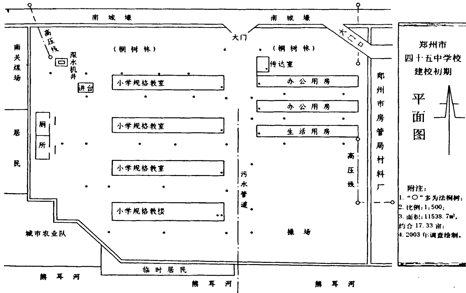
平面图(一)
