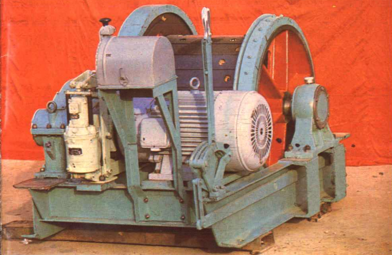
J T 800 提升绞车
