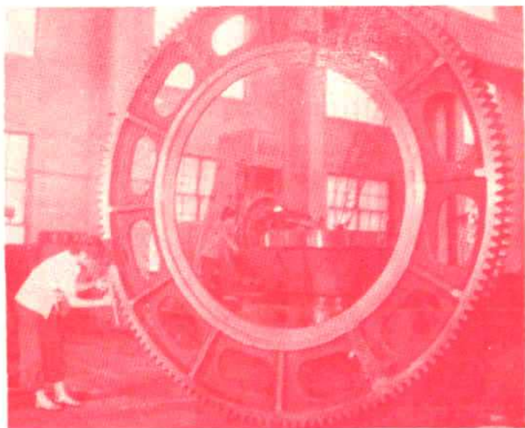
磨机大齿轮在检验
