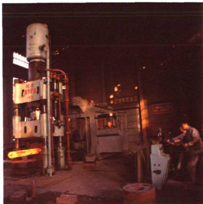
五百吨锻造水压机
