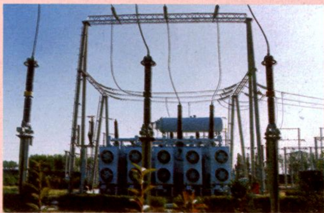
阳高 220 千伏变电站 130000 千伏安主变
