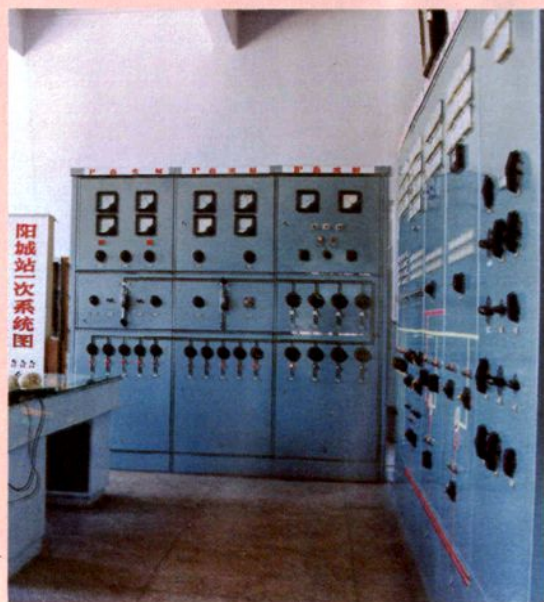
城关 110 千伏变电站主控室
