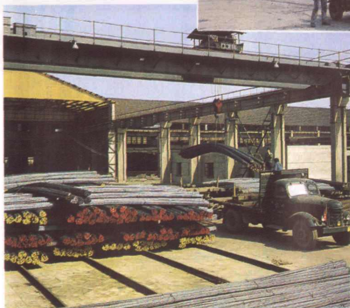
深受用户欢迎的 小型圆钢装运出厂
