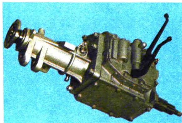
↑ SQC6020A 变速器总成
