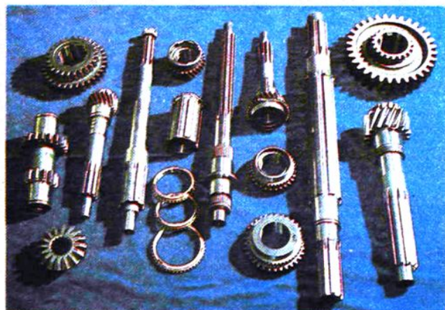
↑ SY132、SQC130、DD680 变速器部份齿轮
