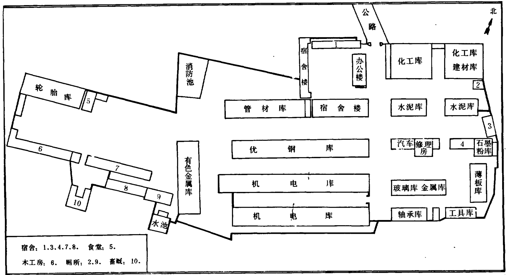
玉溪地区物资局魏家山库区平面图 (1989年)
