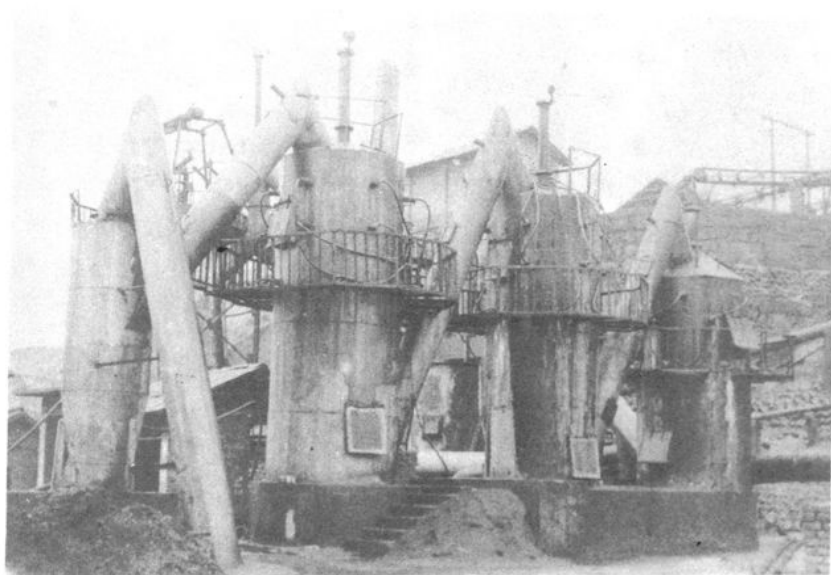
浙江磷肥厂氟硅酸钠吸收系统。
