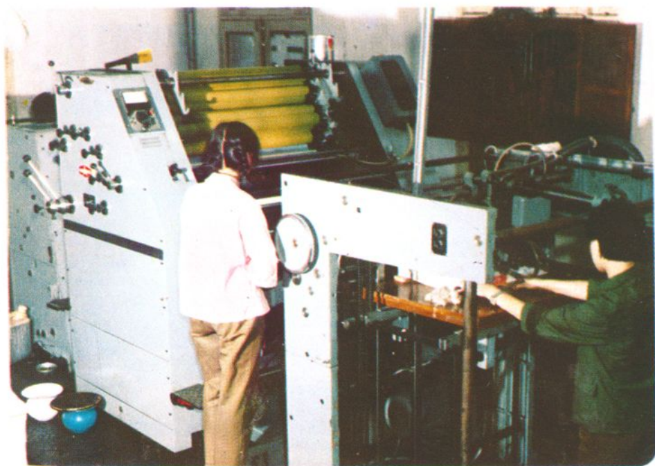
彭县印刷厂08对开胶印机
