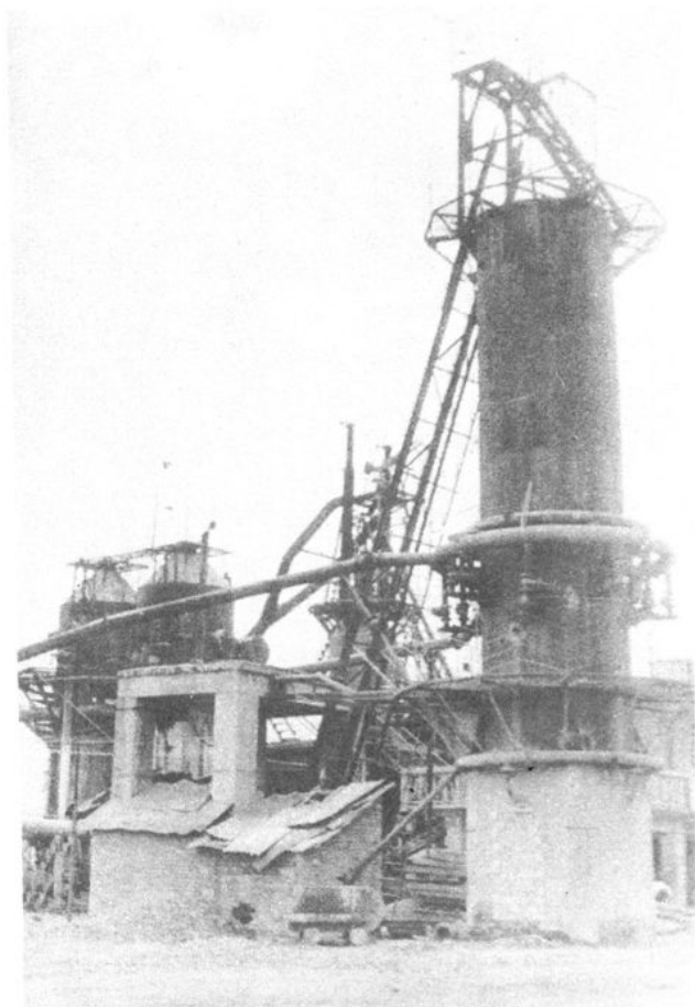
彭县铁厂利用高炉剩余煤气培烧石灰 的18立方米竖炉1981年10月曾获温江 地区工业局节约能源奖。
