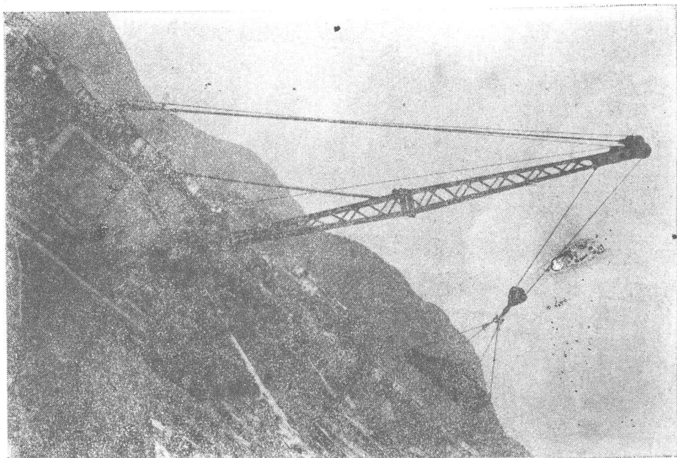
②⑥ ↑ 六都港码头机械五吨吊
