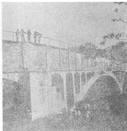
黑龙潭水库黄连咀渡槽
