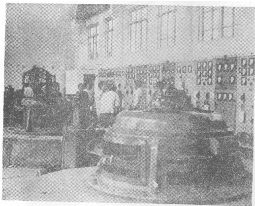
灌县徐渡公社水电站厂房内景
