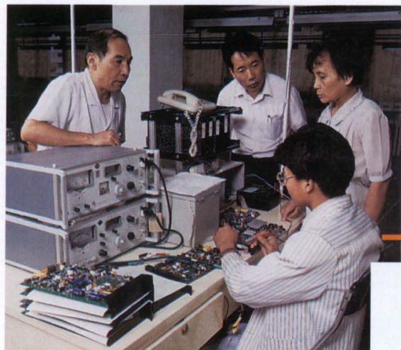
邮科所技术人员在检查T-8用户环路载波机生产情况（1990年）
