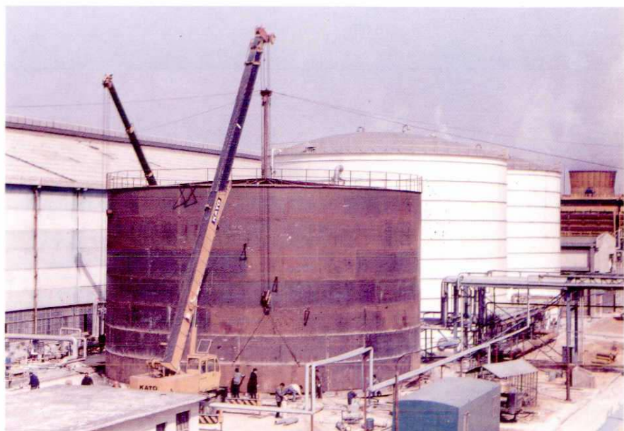
氯碱厂5400m 3 成品罐施工
