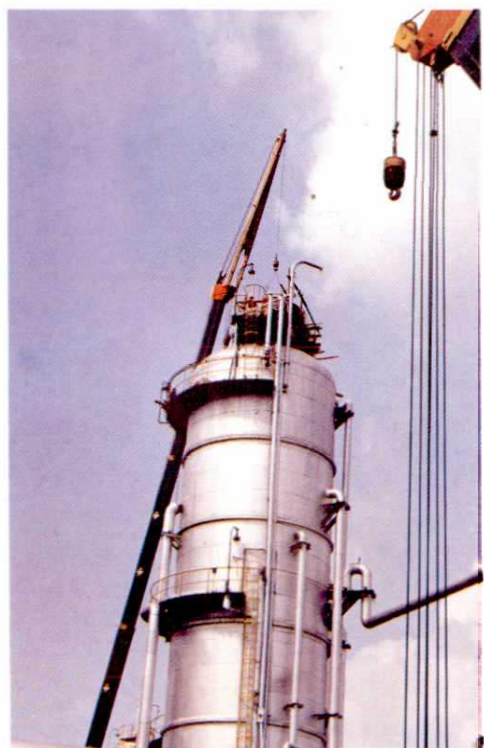
烯烃厂E塔吊装
