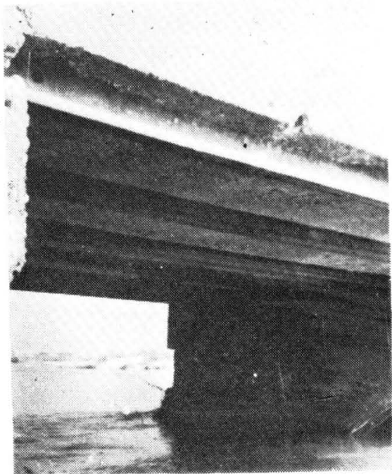
钢轨混凝土梁底面 照片—20（见212页）
