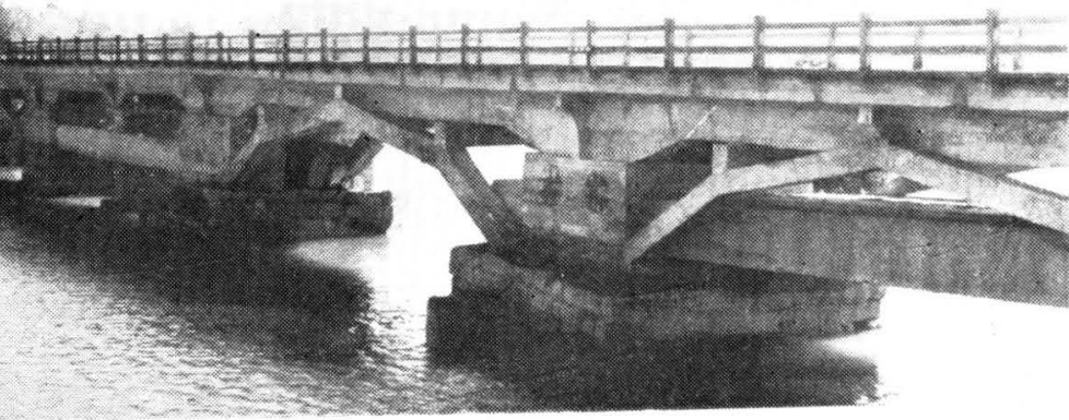
民国时改建的江东桥 照片—18（见205页）
