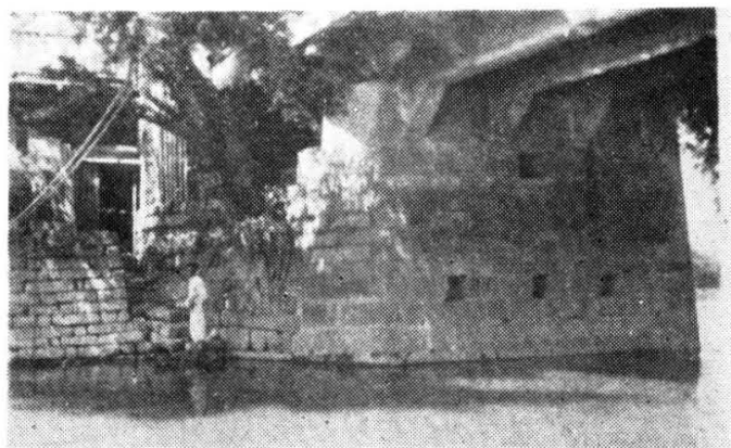
漳州中山桥预留的爆破孔 照片—15（见139页）
