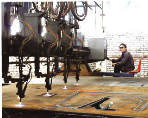
员工操作数控火焰切割机
