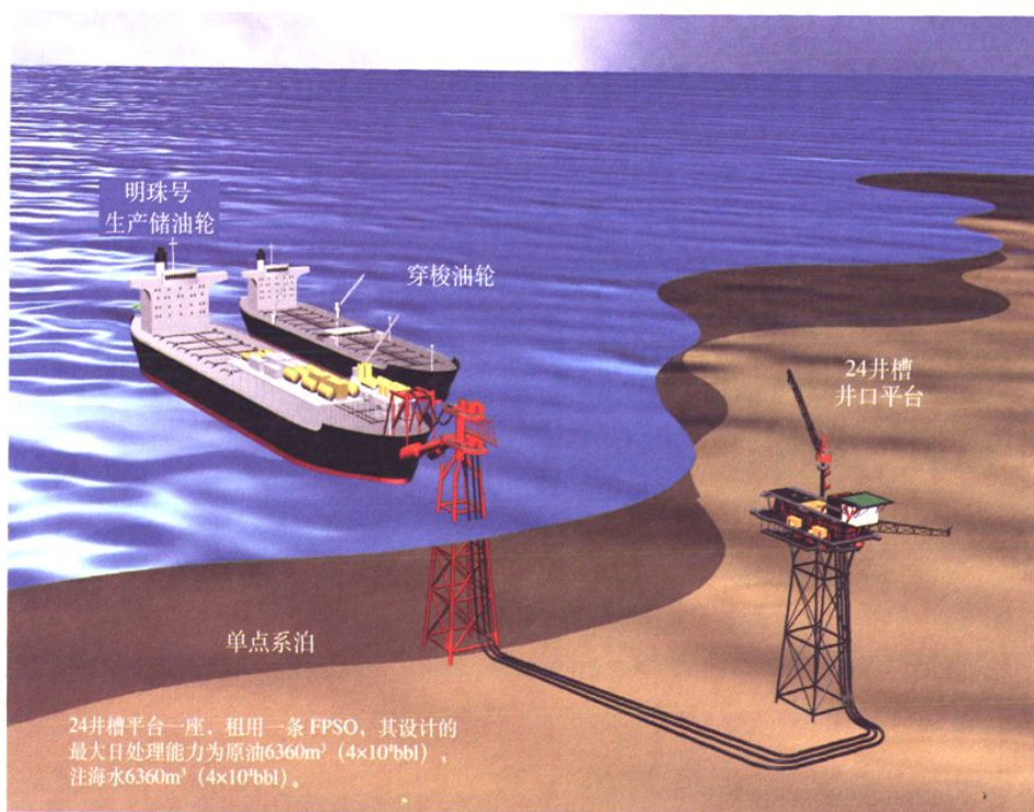
蓬莱 19-3 油田一期地面流程图 (蓬莱 19-3 油田一期 ODP, 2000 年)
