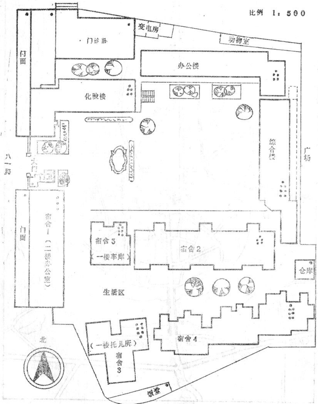
图2 柳州市卫生防疫站总平面布置图
