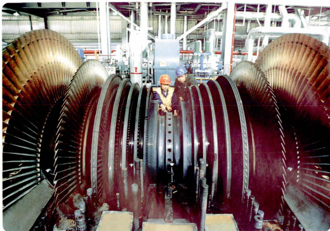
300 MW汽轮机检修现场
