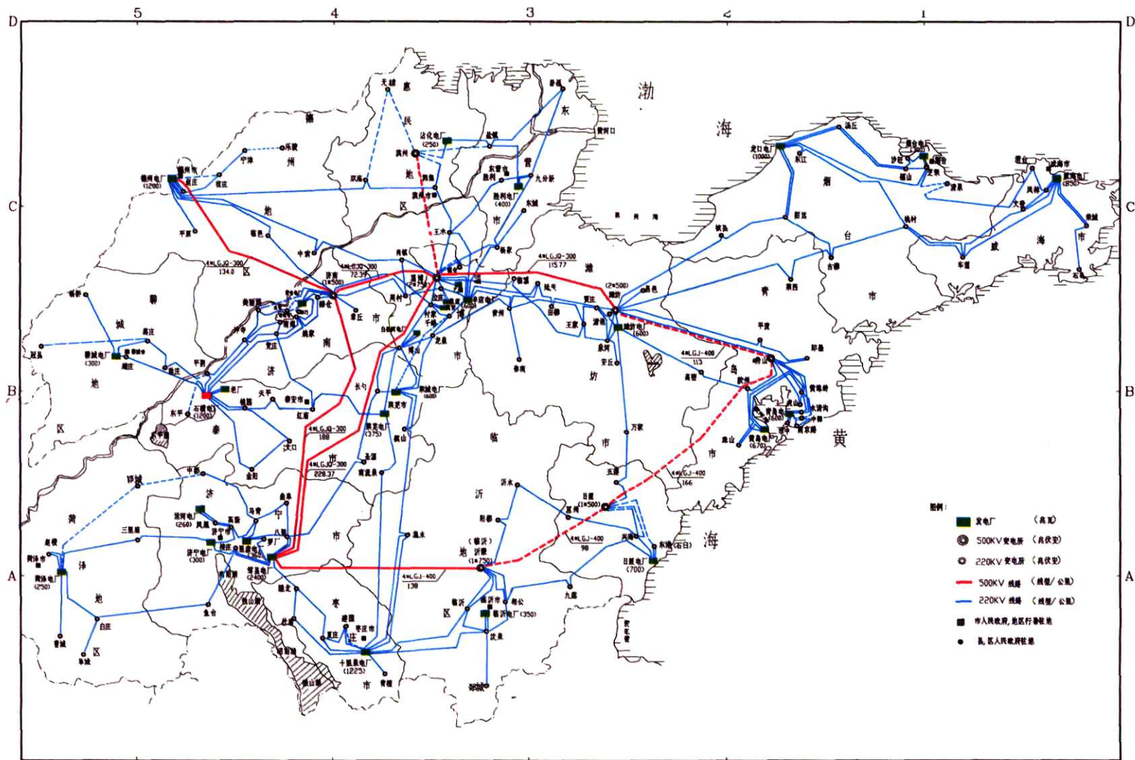
山东石横发电厂与山东电网接线图
