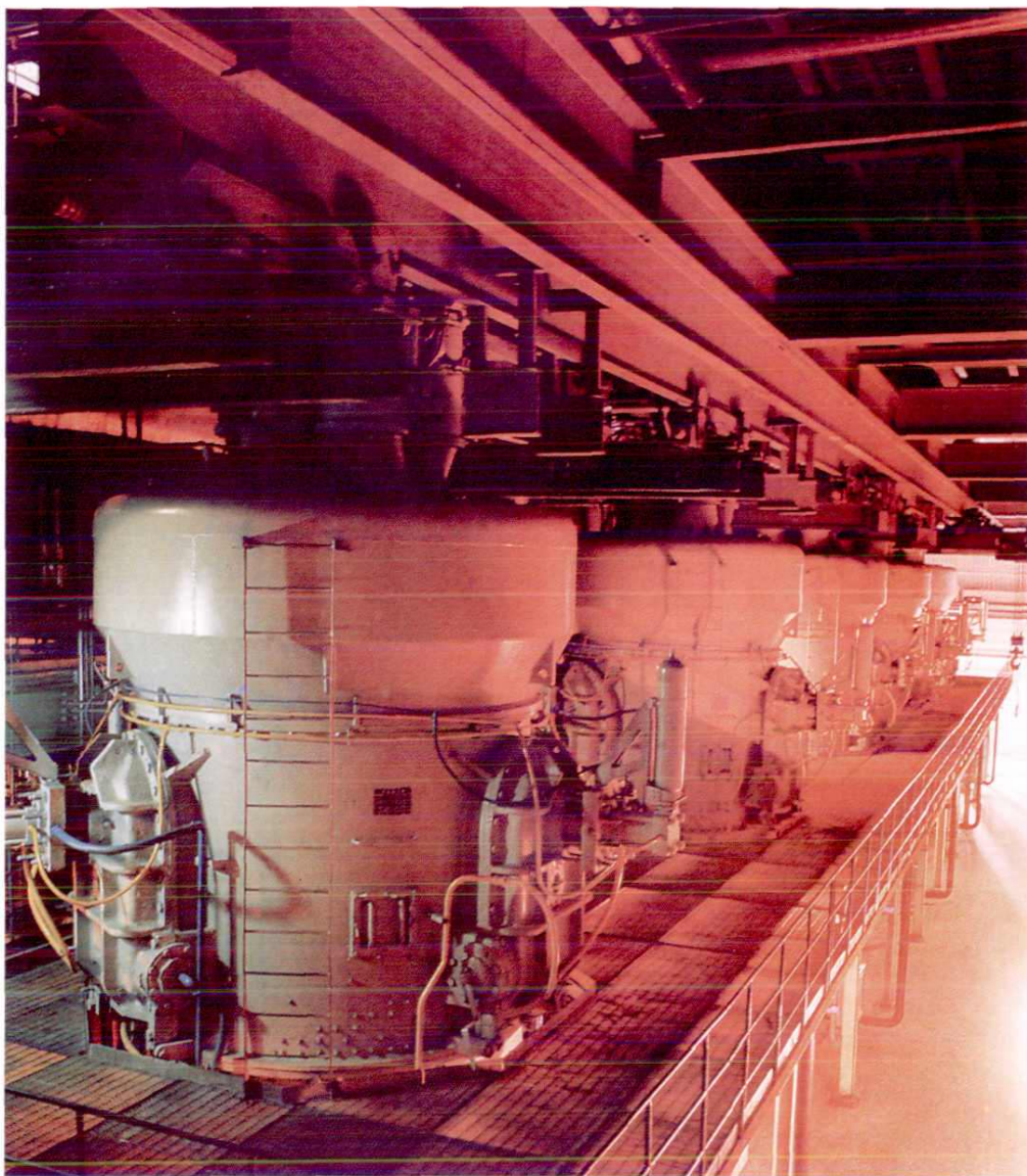
一尘不染的磨煤机房
