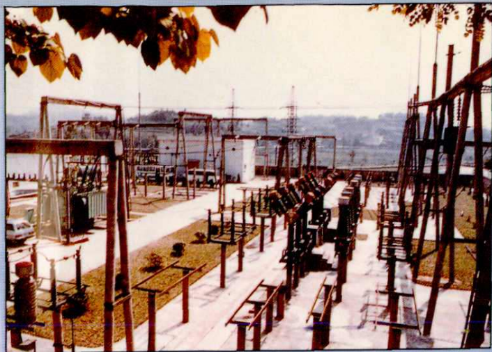
◀ 110 千伏输变电工程
