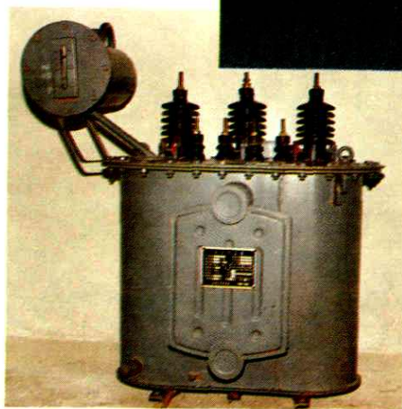
县电机厂生产的节能变压器
