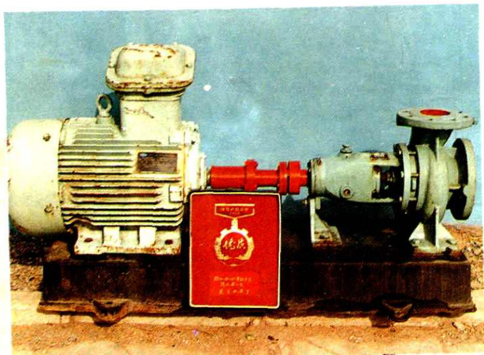
县水泵厂生产的单级单吸清水泵
