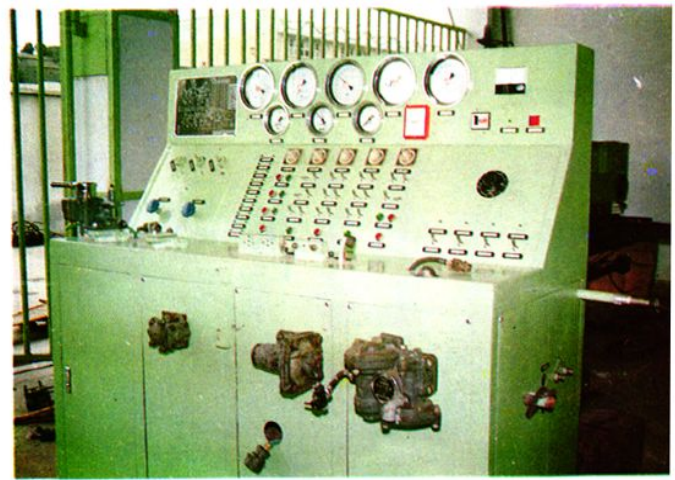
自行研制的DK 1 试验台
