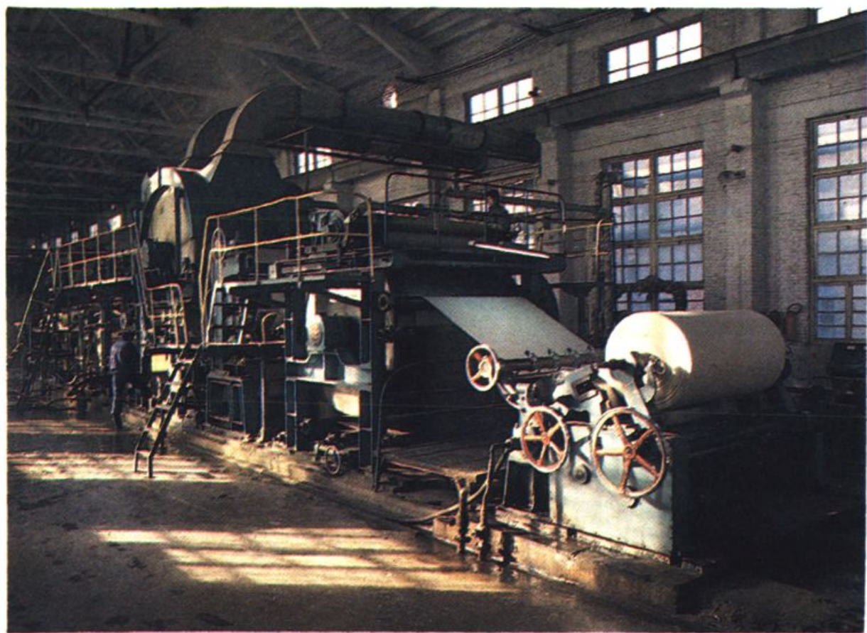
▲ 该厂自行设计生产的ZL2—1760双缸双网造纸机
