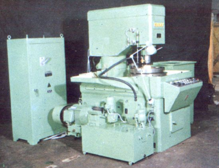
MB4363 B双盘研磨机
