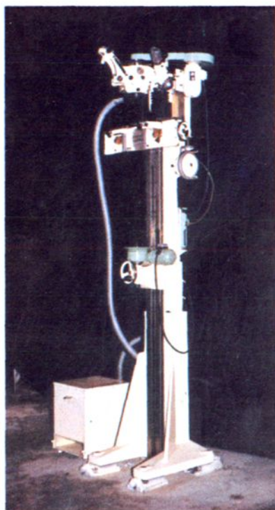
2 M8015 × 2000立式中心孔磨床
