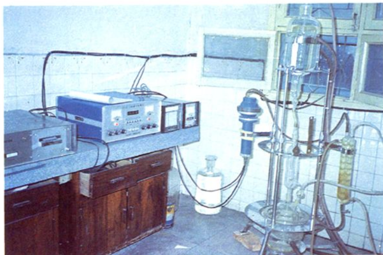
利用温泉进行监测预报地震。图为福建省地震局水化学中心实验站。
