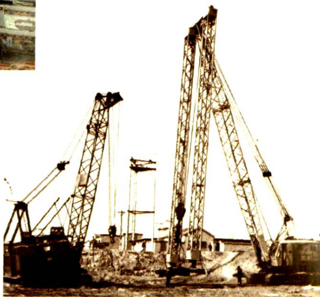
一期工程施工现场
