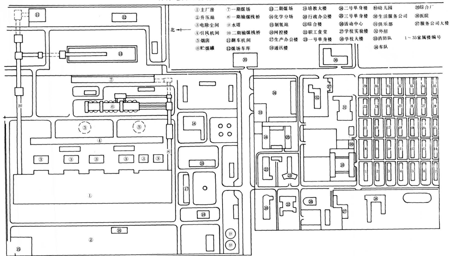
漳泽电力股份有限公司总平面布置图
