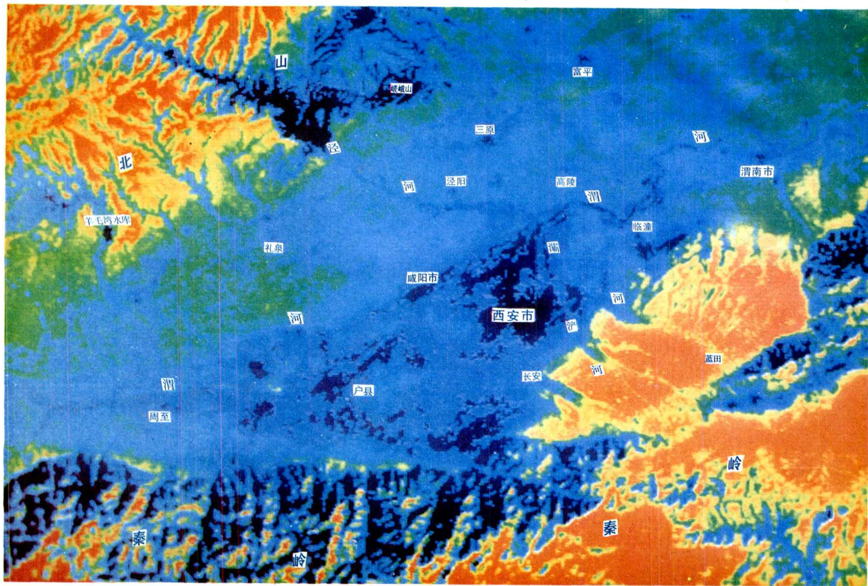
西安地区卫星影像假彩色密度分割图
