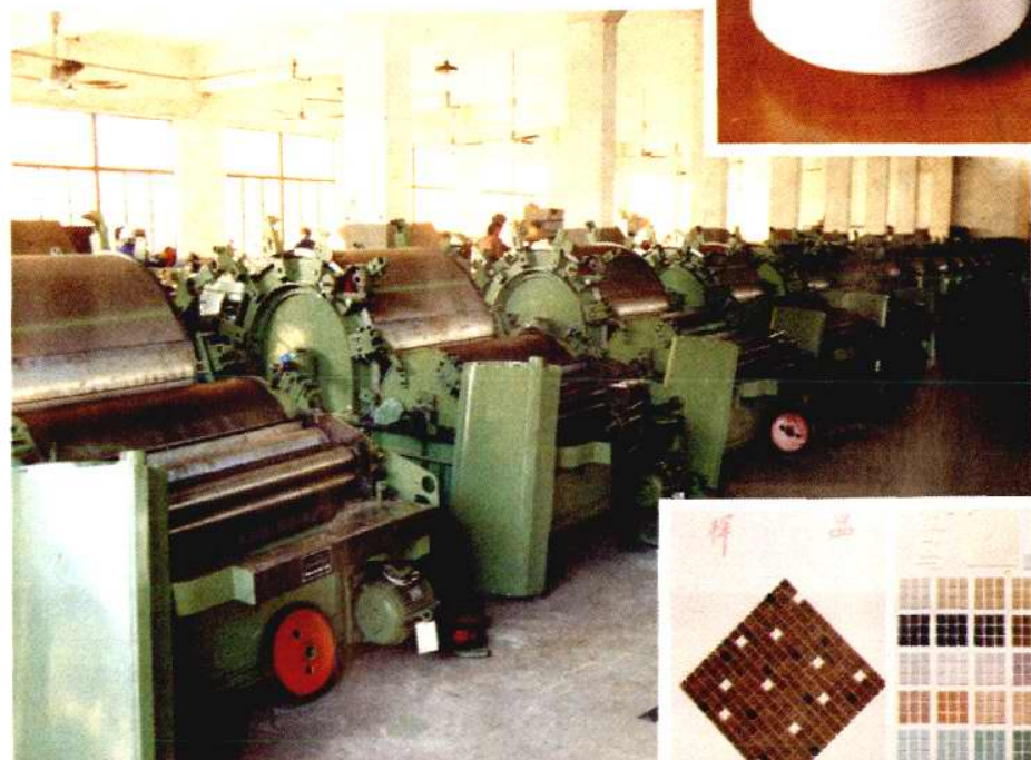
▲ 闽新纺织机械厂生产的梳绵机产品。
