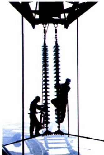
（●）1995年220千伏榕江大跨越工程在进行封航跨江架线。
