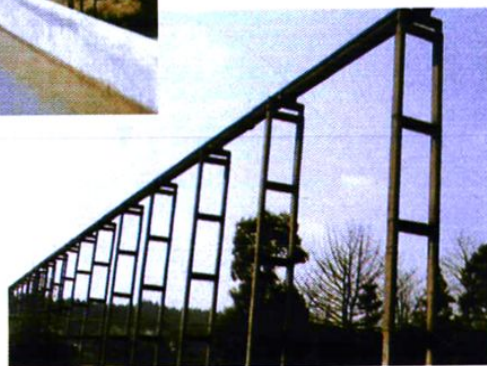
酒埠江灌区东干渠引水渡槽。
