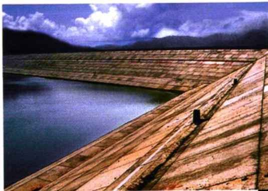
湖南省官庄水库大型砼护坡工程（除险加固工程）。
