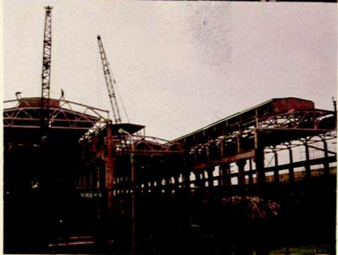
正在兴建的总装工房
