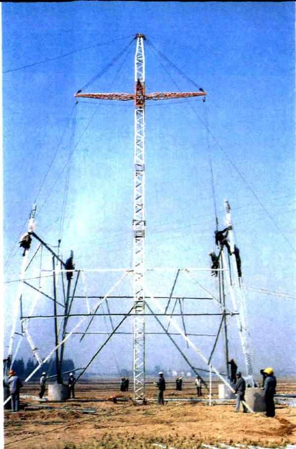
金华电业局送变电工程公司采用通天扒杆组立高塔
